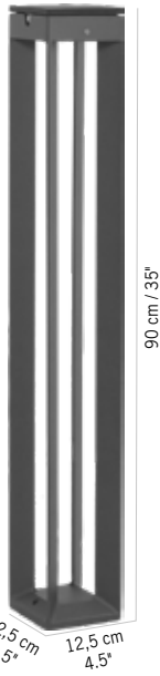
BORNE BLADE À FIXER BLADE pathway light to fix
